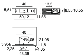
Foratura antina / Door machining
