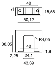
Foratura ripiano / Shelf machining
