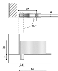
CF0305P / B0 Per vetro spessore mm 6 For glass 6 mm thick
