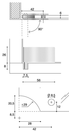
CF0305P / B0 Per vetro spessore mm 6 For glass 6 mm thick
